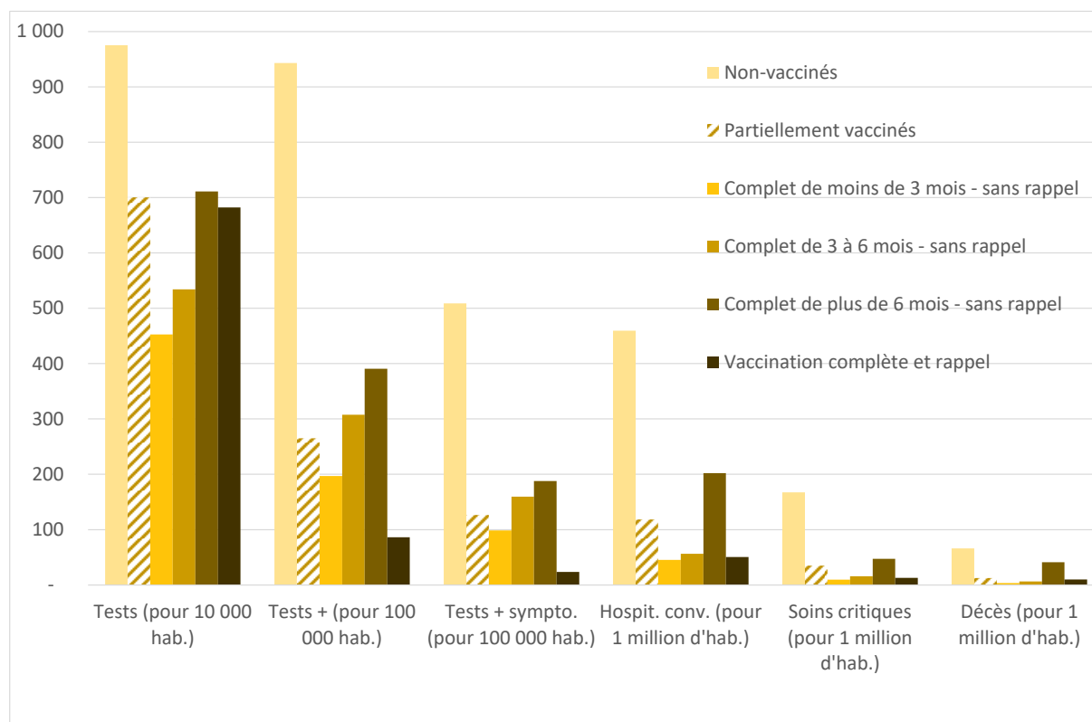
Graphique 2 : Nombre de tests PCR et d'événements hospitaliers à taille de population comparable par statut vaccinal
